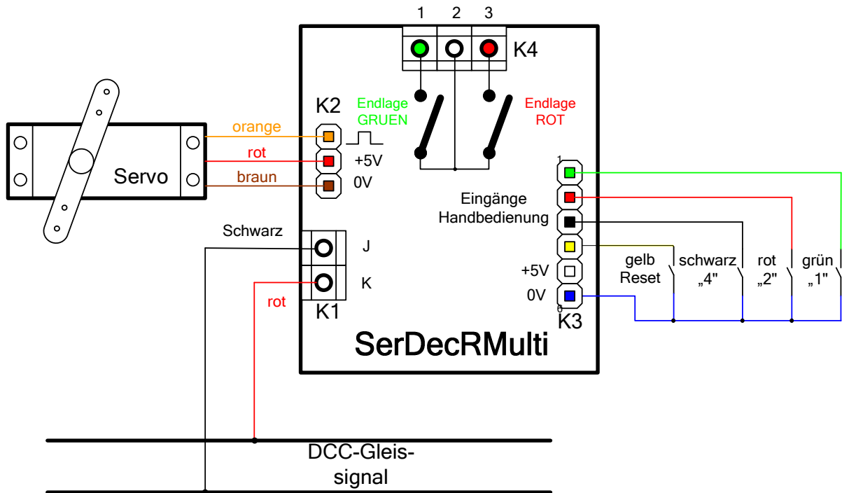
Abbildung 3 – Anschlüsse des SerDecRMulti
