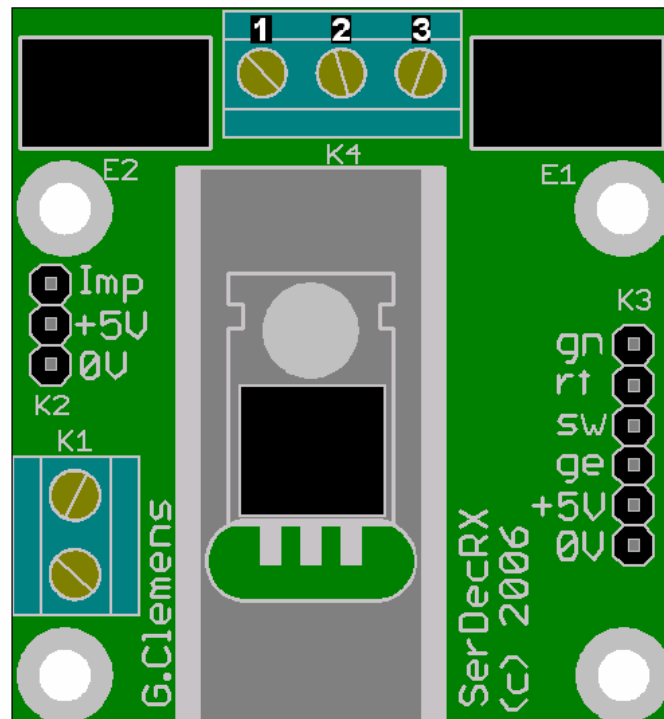
Abbildung 4 – Die Variante SerDecRMulti mit der Lage der Relais E1 und E2 und der Klemmleiste K4 .
