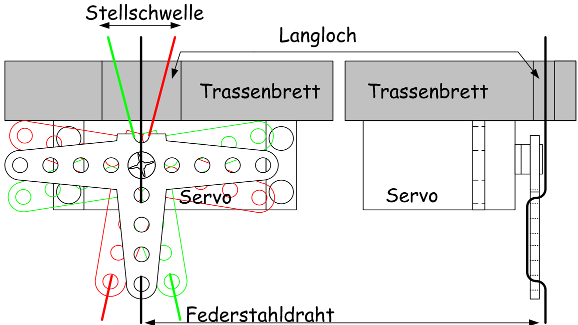
Abbildung 2 – Montage des Servoantriebs unter einer Weiche
