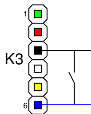
Abbildung 5 – Pfostenleiste K3 mit Brücke/Taster zur Einstellung der Ausgangsadresse
