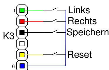
Abbildung 6 – Pfostenleiste K3 mit den Tasten zum Programmieren der Endlagen
