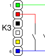
Abbildung 7 – Pfostenleiste K3 mit Tastern für die Handbedienung
