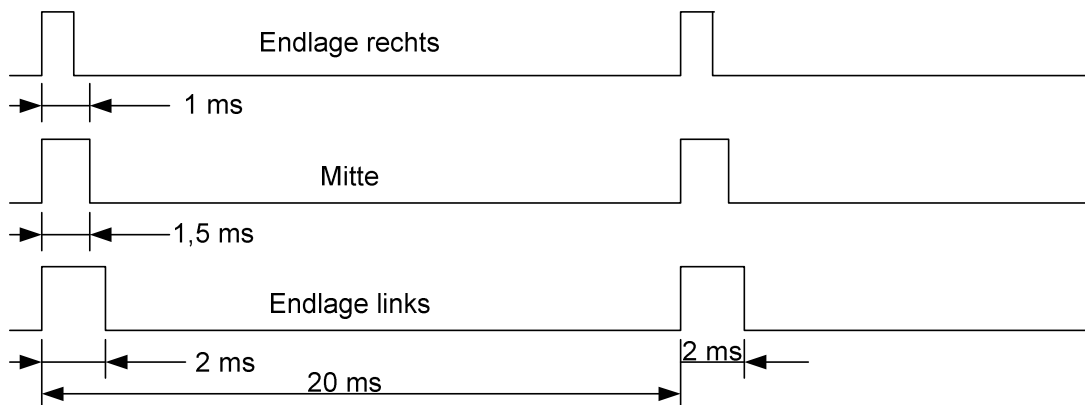
Abbildung 4 – Das Timing des Servosignals
