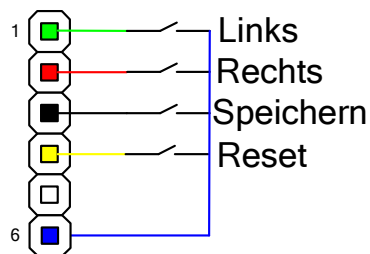
Abbildung 9 – Pfostenleiste mit den Tasten zum Programmieren der Endlagen
