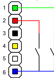
Abbildung 10 – 6-polige Pfostenleiste mit Tastern für die Handbedienung
